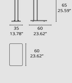
TAPA DE MADERA WOODEN TOP
