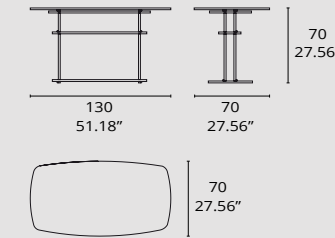
TAPA DE CRISTAL GLASS TOP
